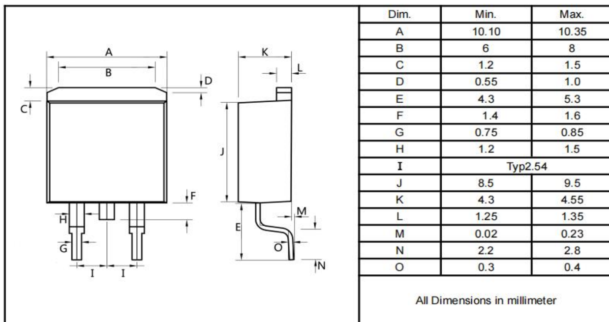
TO-263
